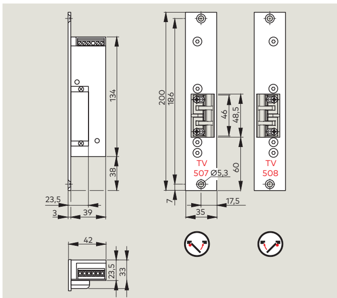
TV 507 / 508 - met schootgeleiding voor stompe deuren
