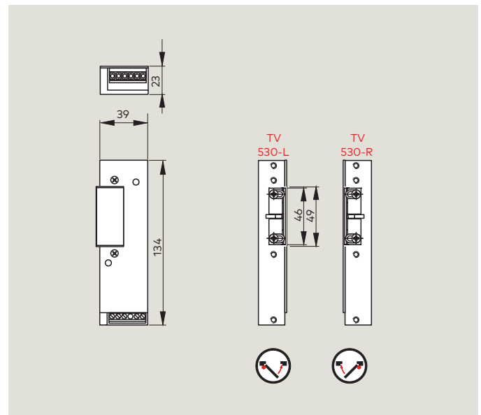
TV 530 - met geïntegreerde terugmeldcontacten
