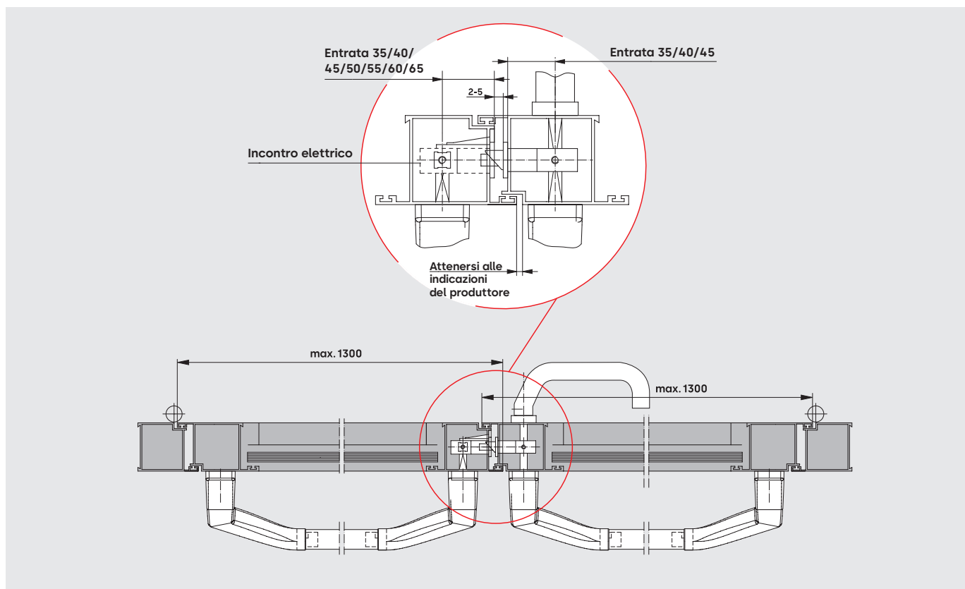
Bloccaggio orizzontale con incontro elettrico montato su una porta con profili in alluminio (Seguire le indicazioni per l'applicazione riportate a pagina 30)
