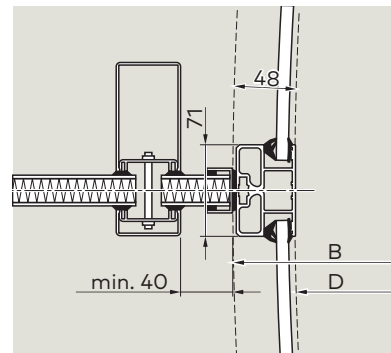
Uitvoering zonder nachtafsluiting
