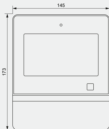
Terminal 96 00, K7-Reihe (Angaben in mm)
