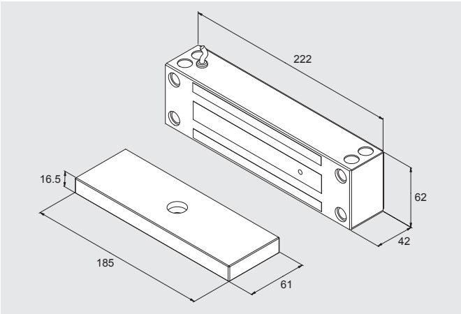
Wymiary dł. x wys. x szer. (mm) Zwora 222 x 62 x 42 Jarzmo 185 x 61 x 16.5
