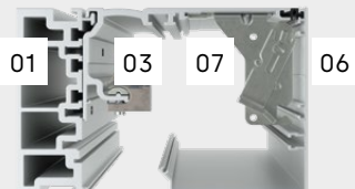
Profiler för korridorinstallation: 120 mm
