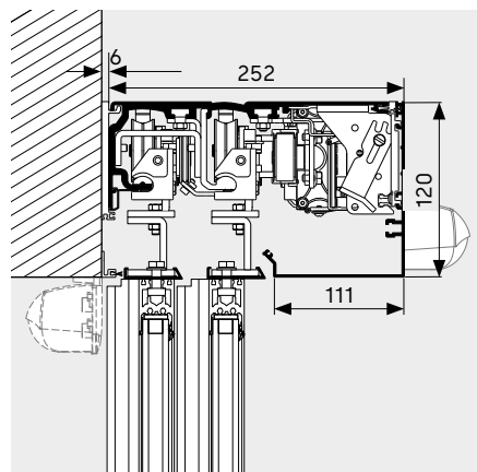
Schematisk illustration av dörrtvärsnitt: väggmonterad, automatikhöjd 120 mm
