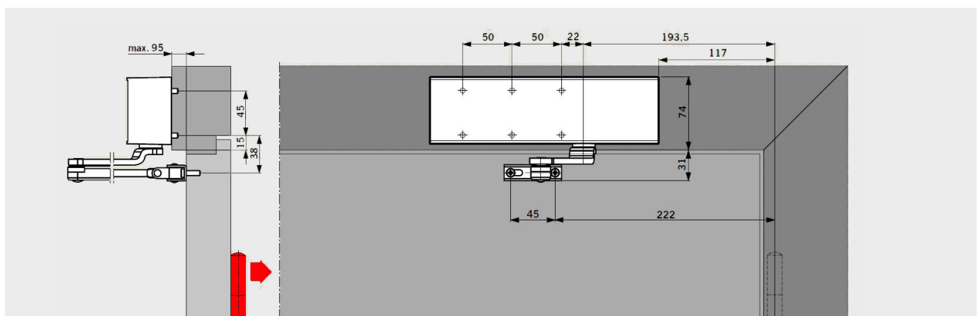
Kozijndorpelmontage aan dagzijde, met normale arm
