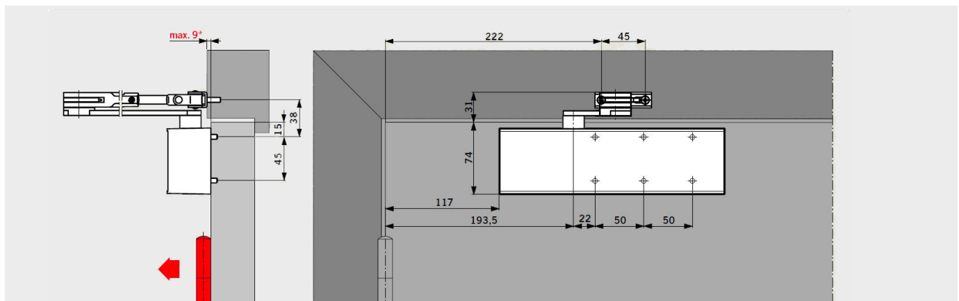
Deurbladmontage aan scharnierzijde, met pal-vastzetarm (Voorbeeld: DIN-linkse deur, DIN-rechtse deur spiegelbeeldig)
