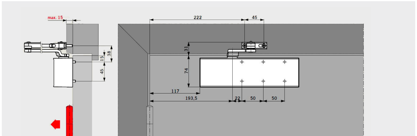
Deurbladmontage aan scharnierzijde, met normale arm (Voorbeeld: DIN-linkse deur, DIN-rechtse deur spiegelbeeldig)
