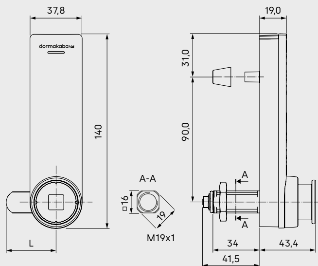
Skabslås 21 20: måltekening forside og side. Mål i mm.
