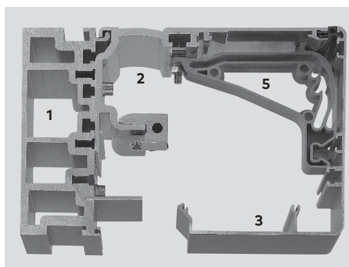
Profielen voor montage in de doorgang 150 mm
