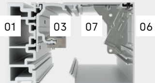
Profiler for korridorinstallasjon: 120 mm
