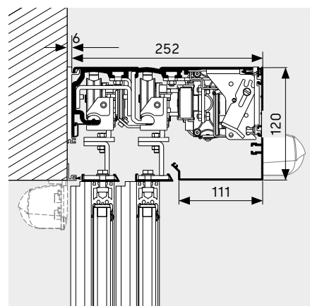
Skjematisk illustrasjon av dørtverrsnitt: veggmontert, drivhøyde 120 mm
