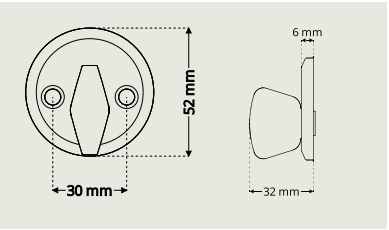
DAK 7330/D7320
