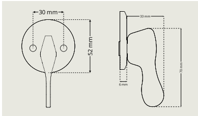
Vrider for nem tilgængelighed
