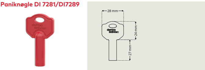
Paniknøgle DI 7281/DI7289
