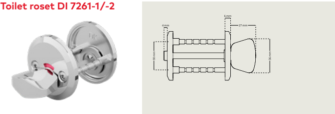
Toilet roset DI 7261-1/-2
