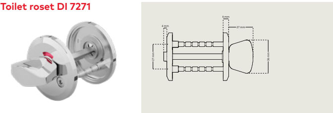
Toilet roset DI 7271
