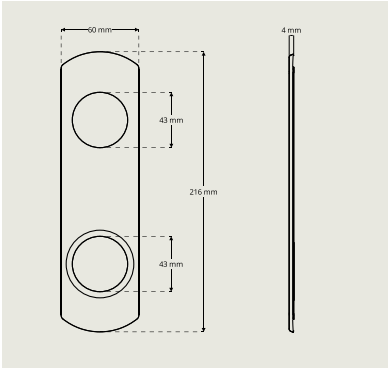
Vrider-roset DA 7200
