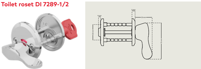
Toilet roset DI 7289-1/2
