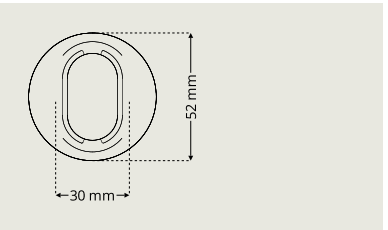
Cylinder roset DR D7320 højder 8-19 mm i samme ring
