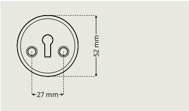
Cylinderskål DA 7395
