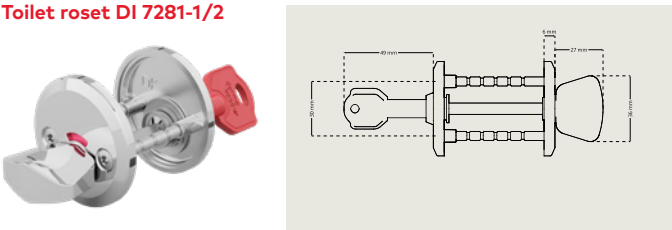
Toilet roset DI 7281-1/2
