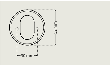
Cylinder roset DR 7320 fås i højder 6-21 mm. Ikke Dynamic.
