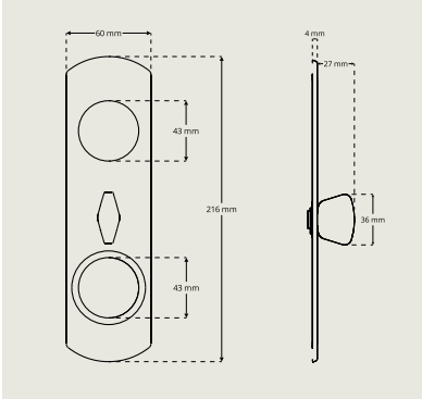
Vrider-dækskilt DP 7709
