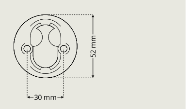
Cylinder roset DR D7330 højder 8-19 mm i samme ring
