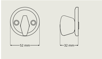
Vrider-roset DA 7200
