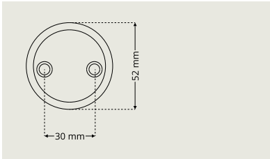
Afstandsring DA 7395
