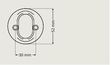
Cylinder roset DR D7320 højder 8-19 mm i samme ring
