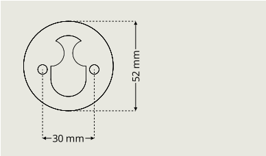
Cylinder roset DR 7330 fås i højder 6-21 mm. Ikke Dynamic.
