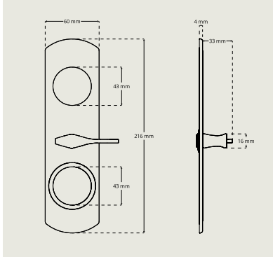
Vrider for nem tilgængelighed
