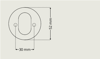
Cylinder roset DR 7340 fås i højder 6-21 mm. Ikke Dynamic.
