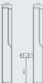
dormakaba leser 90 04, Sidevisning med kabelutgang
