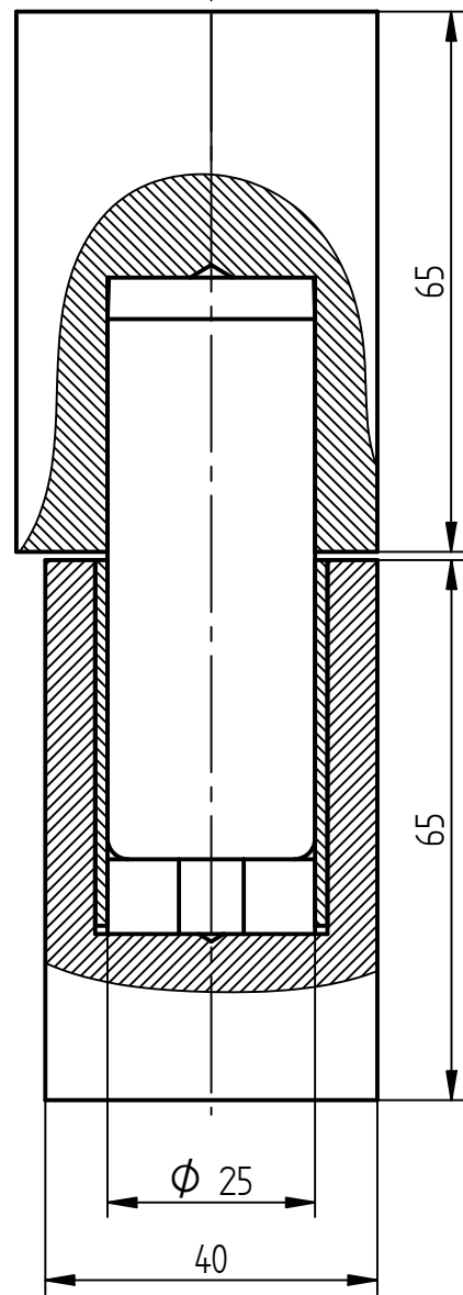
SCHNITT A-A
