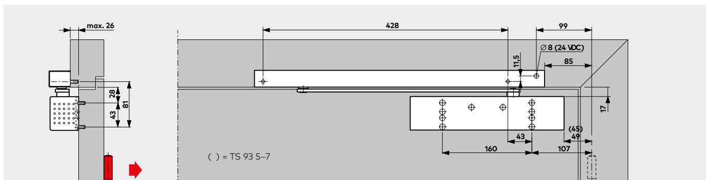
Türschliesser TS 93 G mit Gleitschiene G-EMF, Montage auf der Bandgegensseite Beispiel: DIN-L-Tür, DIN-R-Tür spiegelbildlich
