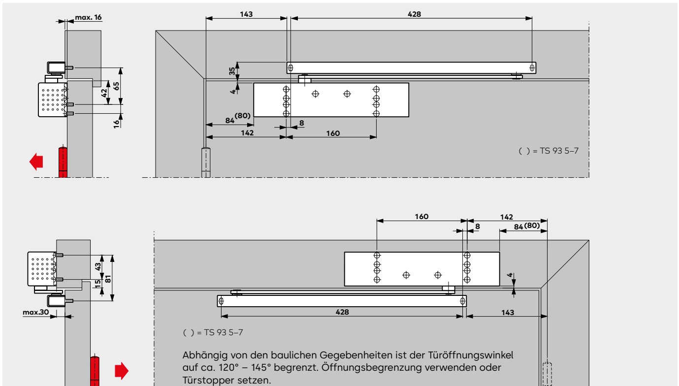
Türschliesser TS 93 B mit Gleitschiene G-N in Türblattmontage auf der Bandseite und Sturzmontage auf der Bandgegensseite Beispiele: DIN-L-Türen, DIN-R-Türen spiegelbildlich
