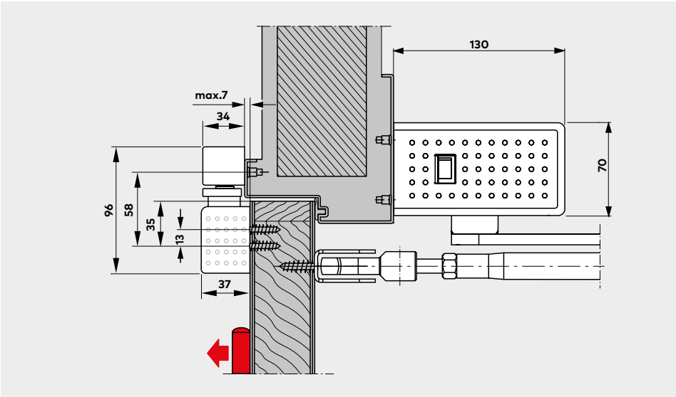
Automatischer Drehflügeltürantrieb ED 100/ED 250 mit Schliessfolgeregler G-SR und G-SR-Drehlager
