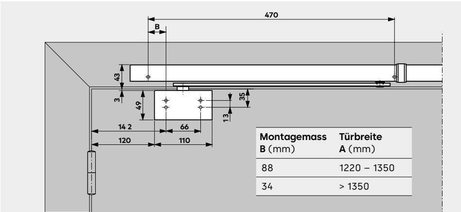
Automatischer Drehflügeltürantrieb ED 100/ED 250 mit Schliessfolgeregler G-SR und G-SR-Drehlager
