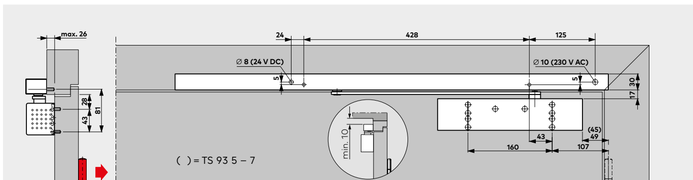
Türschliesser TS 93 G mit Gleitschiene G-EMR, Montage auf der Bandgegensseite Beispiel: DIN-L-Tür, DIN-R-Tür spiegelbildlich
