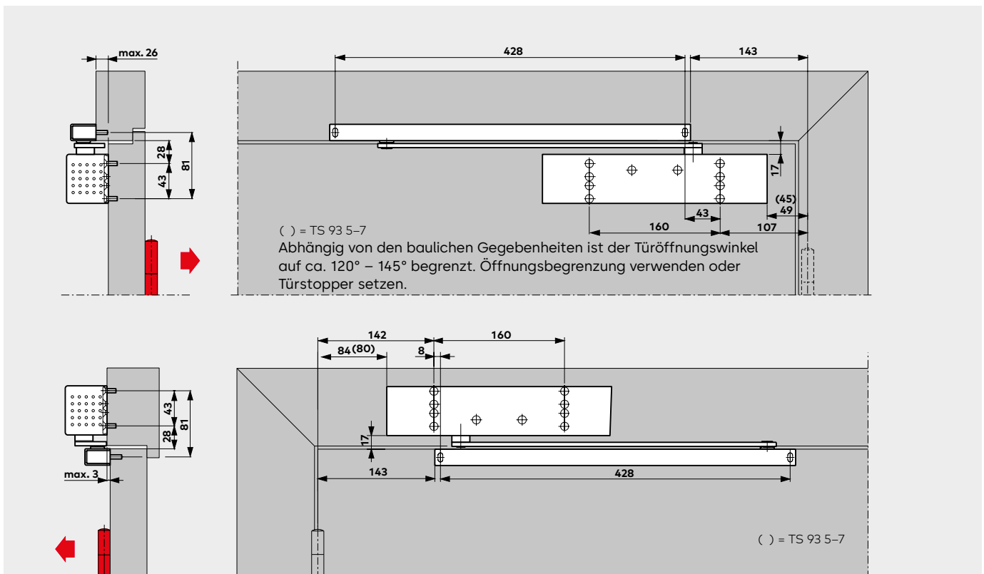
Türschliesser TS 93 G mit Gleitschiene G-N in Türblattmontage auf der Bandgegensseite und Sturzmontage auf der Bandseite Beispiele: DIN-L-Türen, DIN-R-Türen spiegelbildlich
