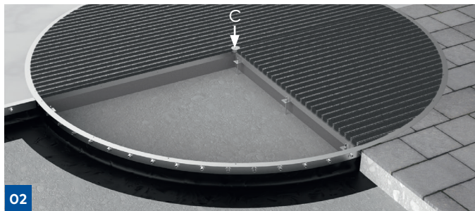
02 Vloerring met klemflens voor aansluiten van folie langs buitenzijde
