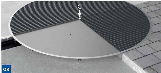
03 Vloerring met waterreservoir voor afvoer regenwater bij slagregen
