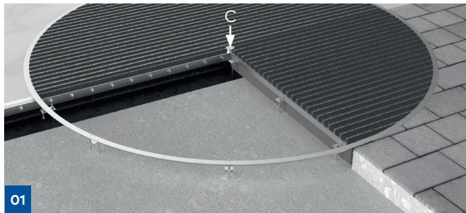
01 Vloerring met klemflens voor aansluiting van folie in de hartlijn
