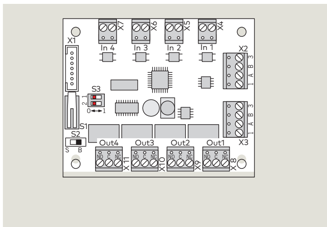
DCW® I/O modul circuitry
