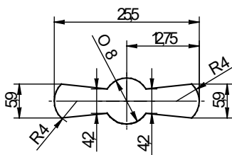
Fig. 1: Key guide 86101
