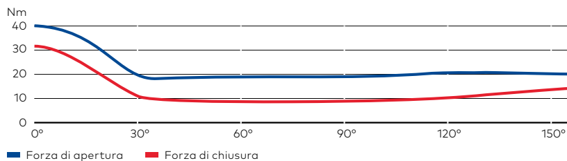
Diagramma dei momenti impostato in EN 4
